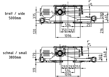
Seitensitz 04 rechts & links mit Armsystem 9.50 Side seat 04 right & left with load booms 9.50
